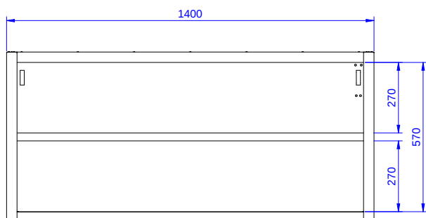
Fronte
